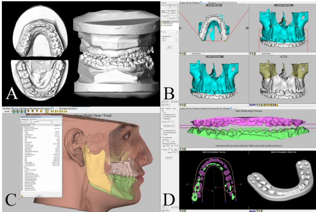
Abb. 1: 3D-Planung eines orthognathen Eingriffs: A) gescannte Gipsmodelle, B) Planung der Le Fort I Osteotomie, C) Simulation der Operation mit Oberkiefer- und Unterkieferverlagerung, D) Design eines 3D-Splints für die Operation
